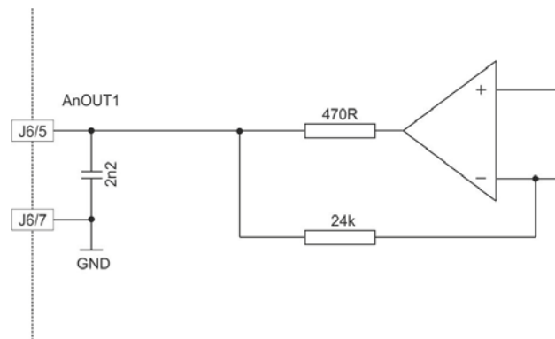
Figure 3-16 Commutation AnOUT1 (dans le principe, s'applique aussi à AnOUT2)
