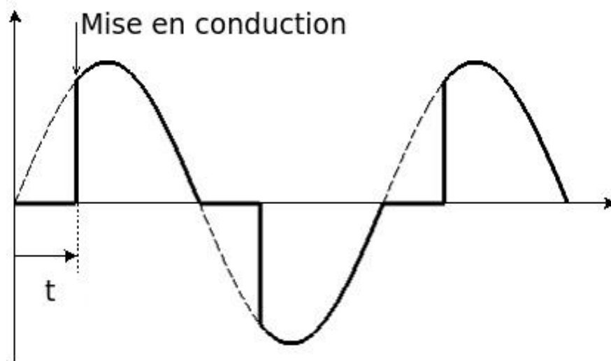
FIGURE 9 – Tension aux bornes de l'ampoule
