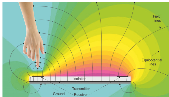
FIGURE 1 – Champ électrique
