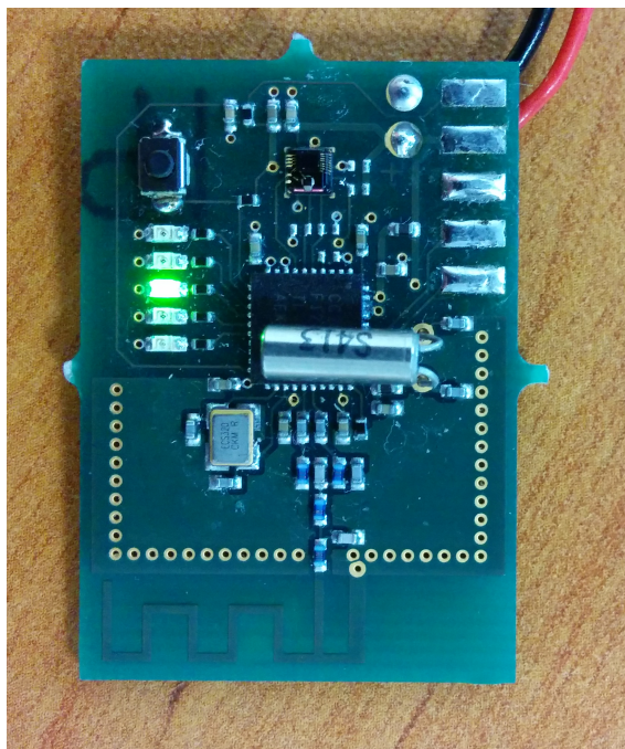
FIGURE 14 – Mode "advertising", attente d'une connexion
