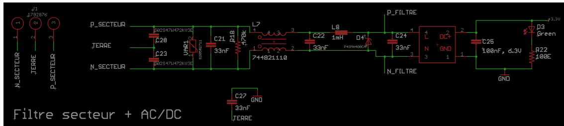
FIGURE 5 – Schéma du filtre secteur
